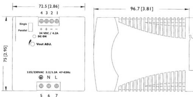
DPP100-24 Dimensions
