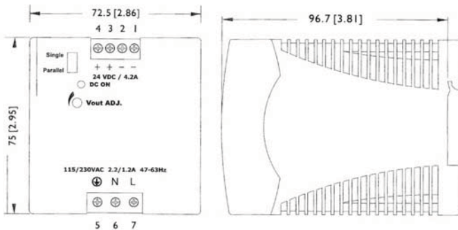
DPP100-24 Dimensions
